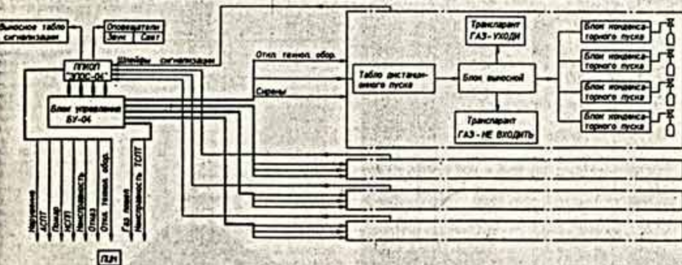
СТРУКТУРА ПОСТРОЕНИЯ КОМПЛЕКСА ТЕХНИЧЕСКИХ СРЕДСТВ «ЭПОС-04 - ПУ-004 СИГНАЛ»
