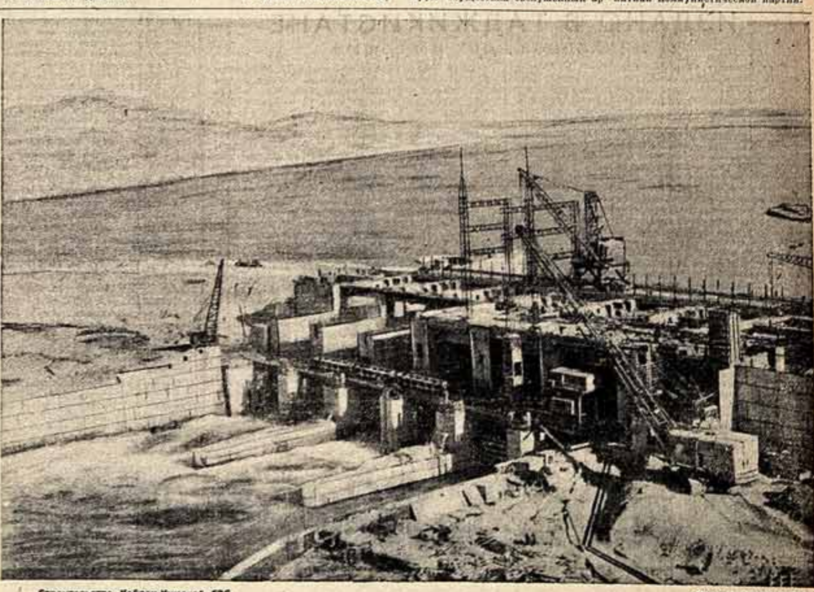
Строительство Байрак-Кумской ГЭС. Фото В. ПИЧУЛИНА.
