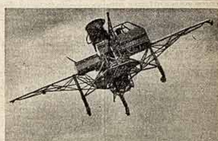
Турболет «Летающий стол» конструкции А. Рафалевича в полете. Фото И. ГАЛАНОВА.
